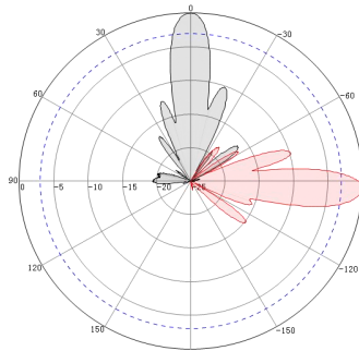
5150MHz
